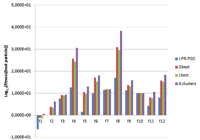
Fig. 8. Dimension 20.
