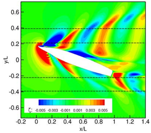
(d) DES 27M
