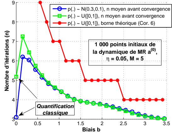
FIGURE 4 – Vitesse de convergence de la dynamique de MR. 1. La convergence est rapide dans les cas extrêmes b petit (quantification classique) / grand (intérêts très divergents); 2. La borne théorique est précise pour b grand.
