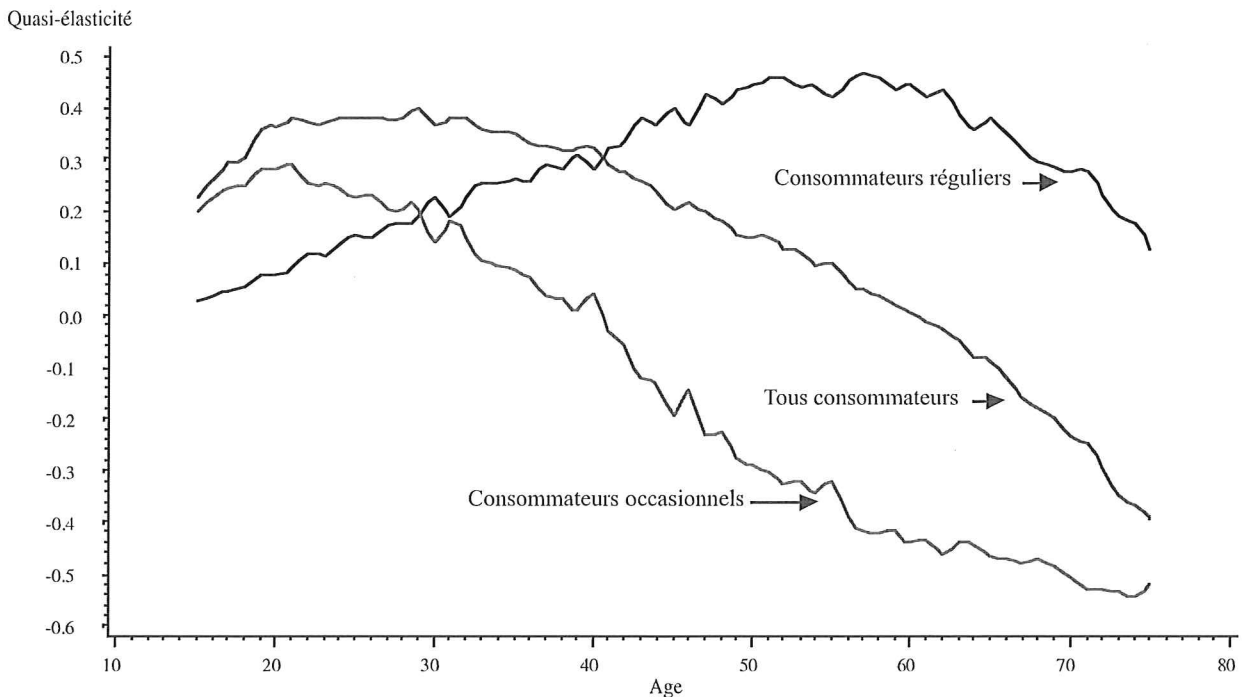
Figure 2. Quasi-élasticités moyennes par âge (calculées à partir du modèle III sur 4010 observations)
