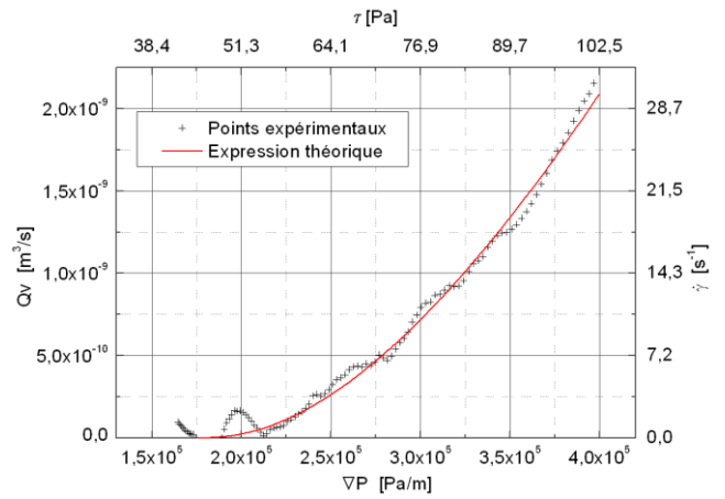
Figure 4 : courbe expérimentale d'injection dans un capillaire unique et niveaux de contrainte et de taux de cisaillement maximaux vus par le fluide.
