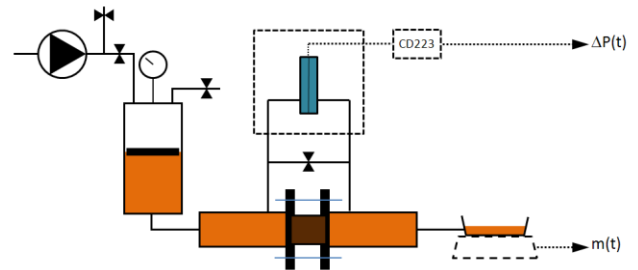
Figure 5 : Schéma du montage expérimental employé
