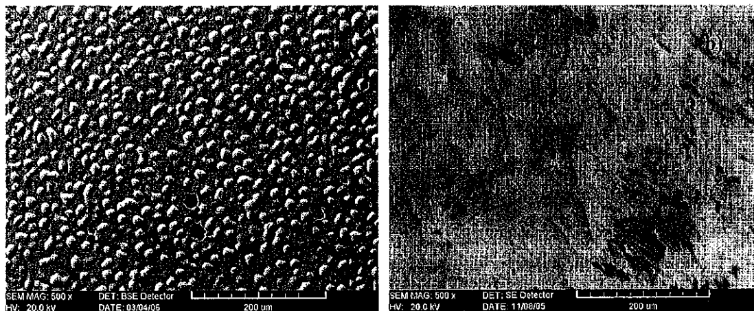
Figure 2 : Micrographie (MEB) : surfaces des films de CrN recuits à 1000°C pendant 1 heure ; t_d = 7.5 mn (-a -), t_d = 90 mn (-b-).
