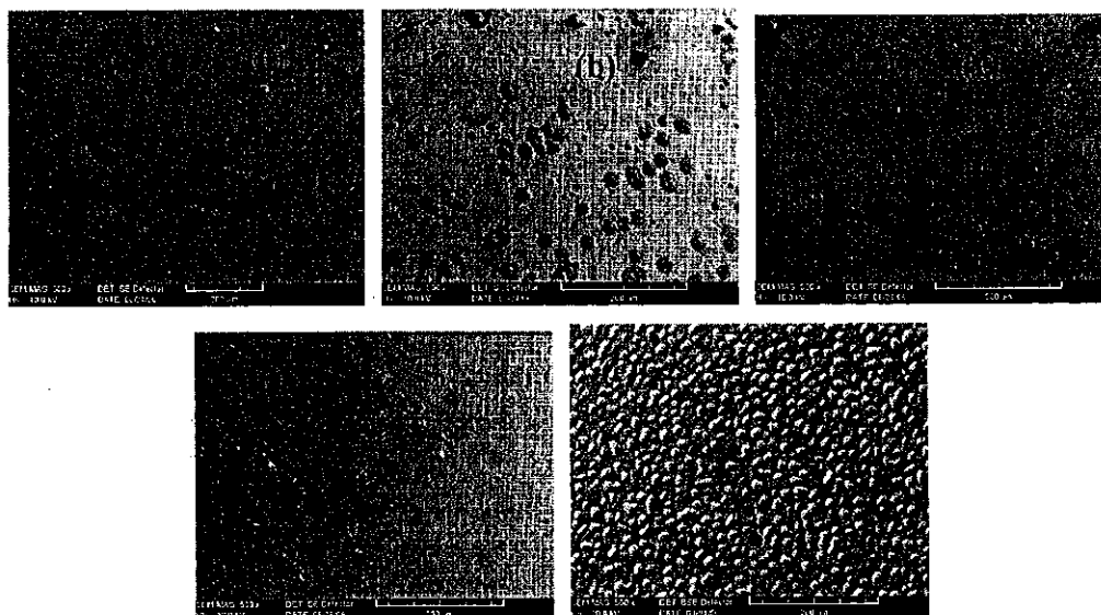
Figure 3 : Micrographies en MEB sur des films CrN à l'état brut (a) et après recuit à 600°C (b), 700°C (c), 800°C (d) et 1000°C (e).
