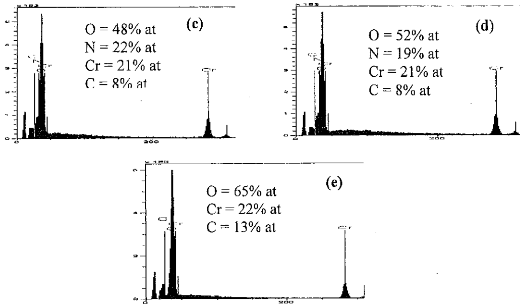
Figure 4: Microanalyses X sur des films CrN ( t_d = 7.5\text{nm} ) recuits pendant 1h sous \text{N}_2 à : 700°C (c), 800°C (d), 1000°C (e).
