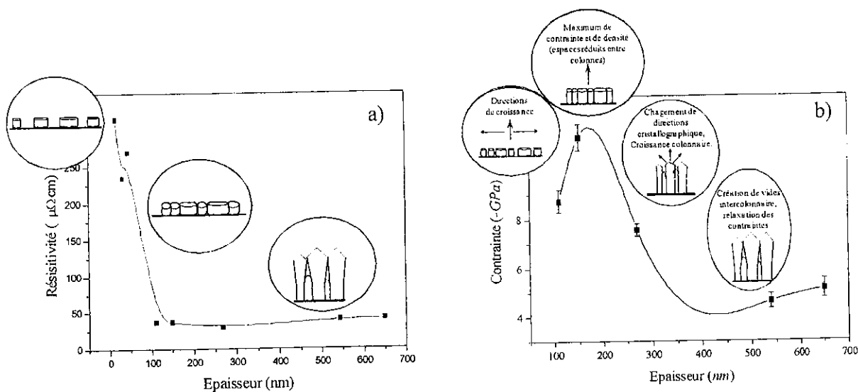
Fig. 5 - Variation de la résistivité (a) et de la contrainte (b) en fonction de l'épaisseur des films
