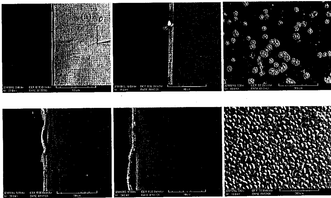
Figure 1 : Micrographies (MEB) des films CrN ( t_d = 7.5 mn) recuits pendant 1 heure à : -600°C {(a) coupe transversale G = 2000x, (b) coupe transversale G = 25000x, (c) surface} -1000°C {(d) coupe transversale G = 5000x, (e) coupe transversale G = 25000x, (f) surface}.
