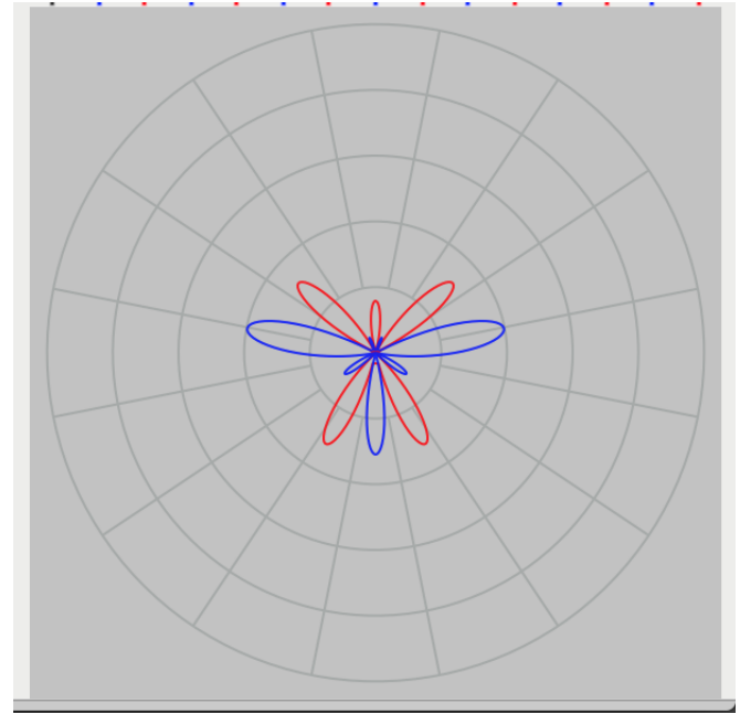
Figure 3. Le facteur de décorrélation est égal à 1. Les harmoniques sont décorréllées, quelque soit le retard appliqué. Le champ est diffus, sa localisation varie de façon très dynamique.
