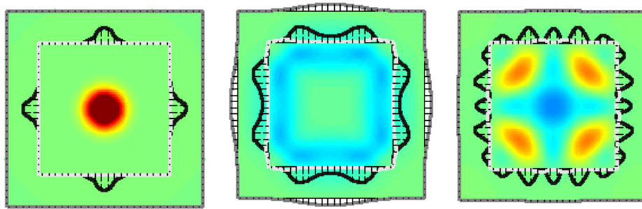
Figure 9. Représentation des taux de restitution dynamiques de l'énergie locaux à différents instants pour une condition initiale hautes fréquences dans la zone molle
