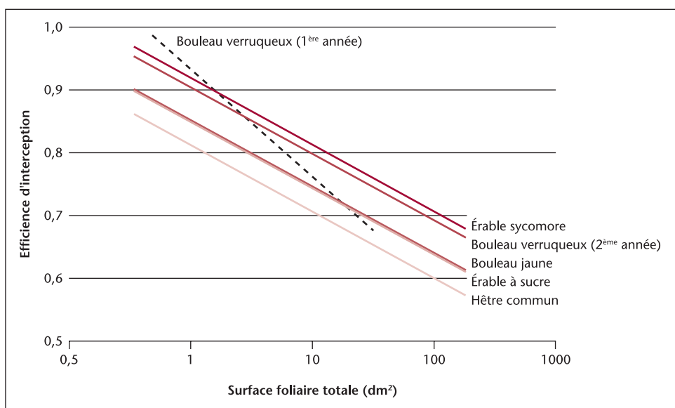
Figure 1 – Efficienc d'interception de la lumière en fonction de la surface foliaire totale de jeunes plants de 1 et de 2 ans cultivés sous différents niveaux de lumière (d'après DELAGRANGE et al. 10 ). Les traitements de lumière n'ont induit aucune différence et ne sont donc pas indiqués. Les différences entre espèces sont significatives. À surface foliaire équivalente, l'efficienc d'interception du hêtre est la plus faible.
