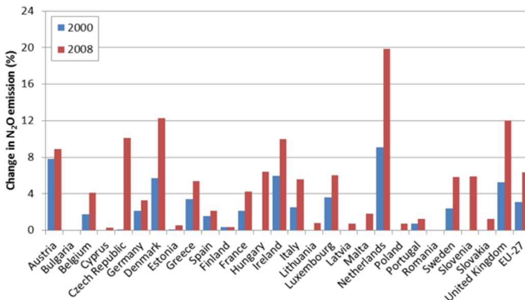
Figure 13 – Variation des émissions de N 2 O entre le scénario « réel » et le scénario « sans directive nitrate »
