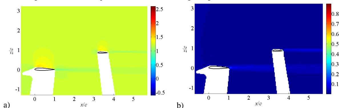
Figure 6 : Écoulement pour l_x = 3,19 c , l_z = c et \alpha = 0^\circ : a) vitesse axiale relative, b) écart-type de fluctuations de vitesse axiale.
