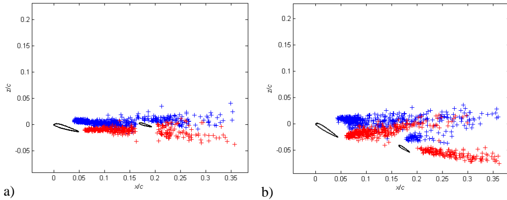
Figure 11 : Trajectoires des LEV (bleu) et des TEV (rouge) des profils pour a) \alpha = 15^\circ , b) \alpha = 30^\circ .
