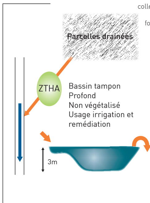
Figure 33 : Schéma de principe des deux types de zones tampons humides artificielles (ZTHA) testés par le Cemagref.
