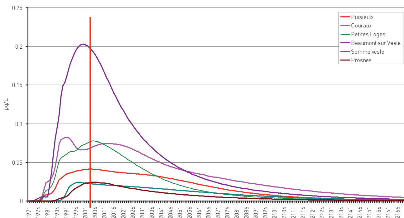
Figure 27 : Simulation des concentrations moyennes annuelles en atrazine entre 1971 et 2170, dans le bassin versant de la Vesle.
