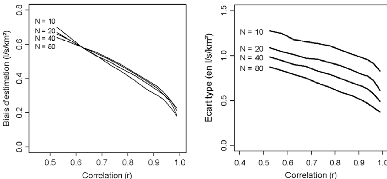
Figure 3 : Exemple d'évolution du biais \mu et d'écart-type \sigma en fonction de la corrélation et du nombre de jaugeages pour une fréquence annuelle de cinq jaugeages
