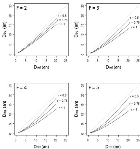
Figure 6 : Durée de suivi équivalente D_{eq} pour F > 1 en fonction de la durée de suivi D_{réf} pour F_{réf} = 1 pour différents niveaux de corrélation
