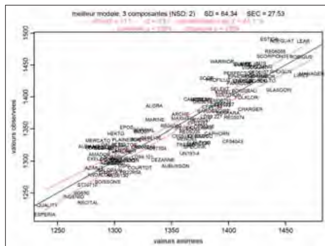
Figure 12 : régression PLS pour expliquer les valeurs moyennes d'épiaison 2009 en prenant comme variables explicatives les allèles aux gènes Vrn1 , Ppd et Ft , et la précocité intrinsèque.
