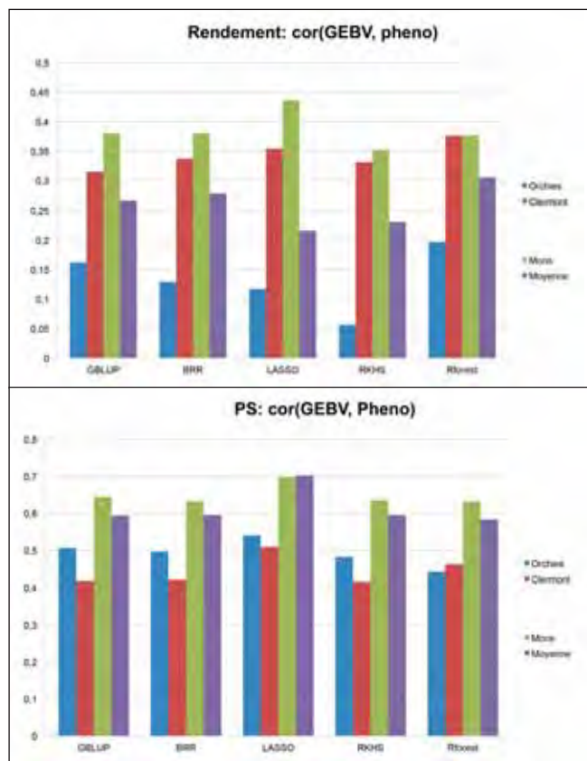
Figure 4 : Efficacité (corrélations entre GEBV et phénotype) par validation croisée pour 5 méthodes statistiques dans les 3 lieux et la moyenne, pour 2 caractères cibles.
