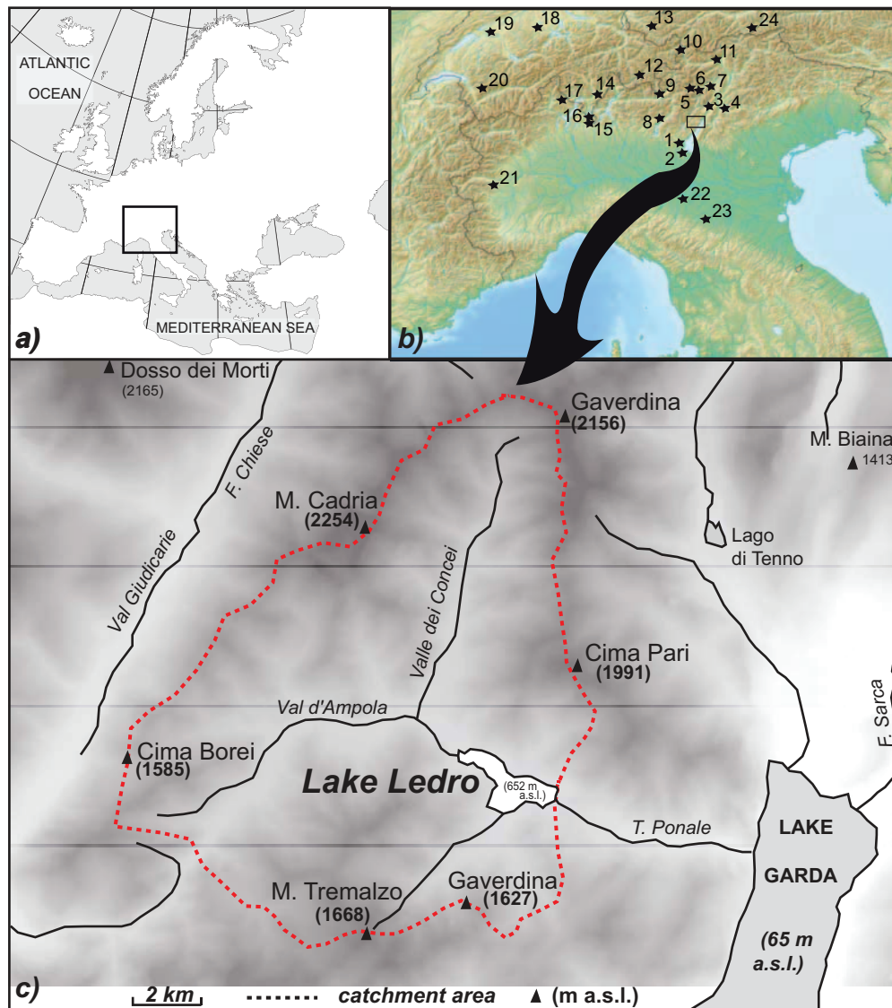
Figure 1. (a) The study site in the Northern Mediterranean area; (b) location of pollen sites discussed in the paper for the Alps and Northern Italy (1: Lake Lucone (Valsecchi et al., 2006), 2: Lake Lavagnone (De Marinis et al., 2005), 3: Fiavé-Carera (Marzatico, 2007), 4: Lake Lavarone (Filippi et al., 2007), 5: Valle di Sol (Favilli et al., 2010), 6: Lago Nero di Cornisello (Filippi et al., 2005), 7: Lake Tovel (Gottardini et al., 2004), 8: Valcamonica (Nash, 2012), 9: Pian di Gembro (Pini, 2002), 10: Ötztal Alps (Festi et al., in press), 11: Totenmoss (Heiss et al., 2005), 12: Lej da San Murezzan (Gobet et al., 2003), 13: Montafon Valley (Röpke and Krause, 2013), 14: Val Febbraro (Moe et al., 2007), 15: Lago di Muzzano (Tinner et al., 2003), 16: Lago di Origlio (Tinner et al., 2003), 17: Piano and Segna (Valsecchi and Tinner, 2010), 18: Soppensee (Tinner et al., 2003), 19: Lobsigensee (Tinner et al., 2003); 20: Lauenensee (Rey et al., 2013), 21: Lago Piccolo di Avigliana (Finsinger and Tinner, 2006), 22: Terramara di Santa Rosa di Poviglio (Cremaschi et al., 2006), 23: Terramara di Montale (Mercuri et al., 2006), and 24: Spannagel Cave (Mangini et al., 2005)); and (c) catchment area of Lake Ledro (dotted line).
