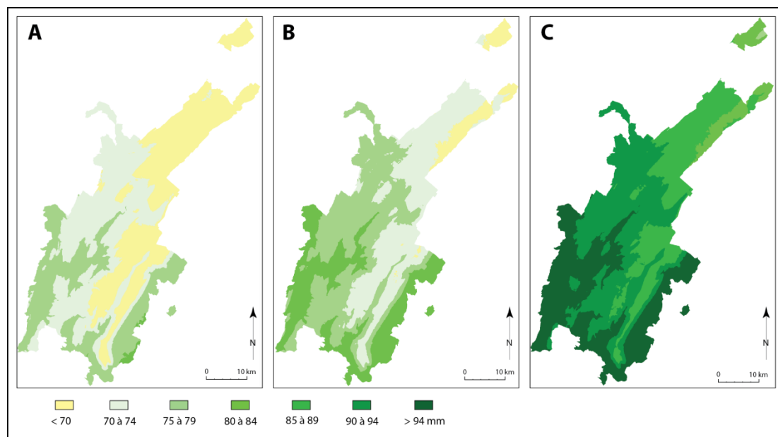
Figure 3.24 : ETP (mm) de juillet pour les trois normales (1981-2010 (A), 2021-2050 (B) et 2071-2100 (C))
