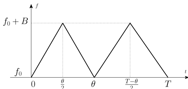
Figure 1. La forme d'onde "FMCW double".
