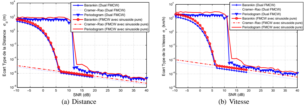
Figure 3. FMCW double et FMCW avec sinusoid pure. Comparaison des performances pour l'estimation de la distance (a) et de la vitesse (b) ( d = 50 m, v = 80 km/h).
