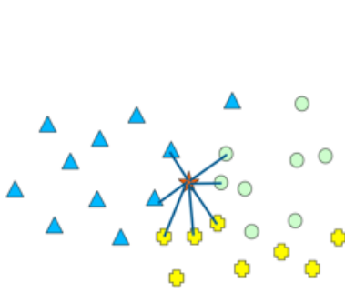
FIGURE 6: Les K plus proches voisins. A quelle classe appartient l'étoile dépend trop du K.
