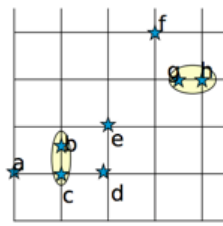
FIGURE 11: Deuxième étape de la CAH. Les données b,c et g,h ont été fusionnées parce qu'elles étaient les plus proches
