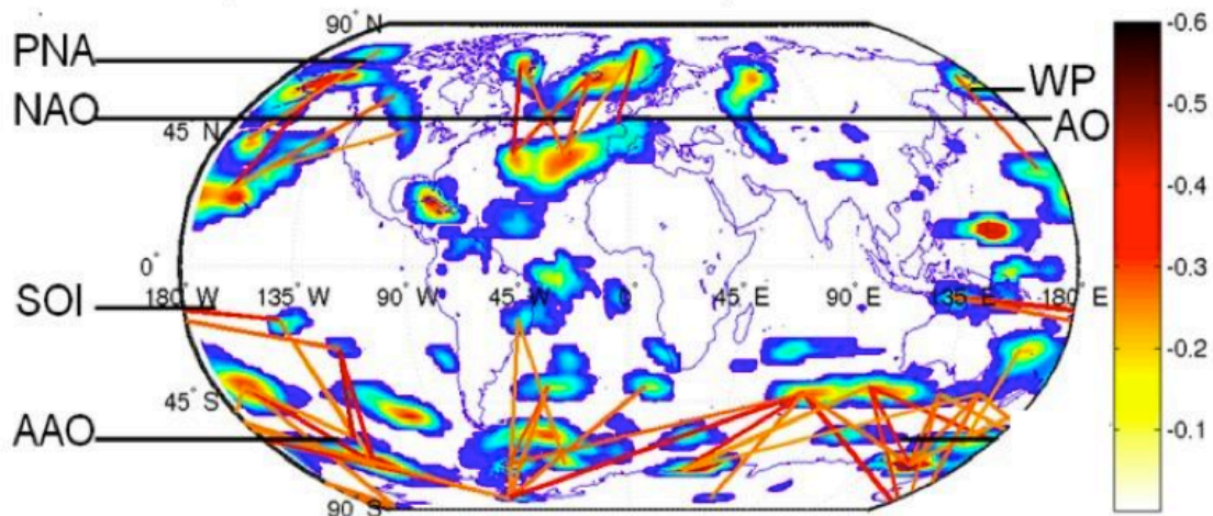
FIGURE 1: Application de la méthode automatique de détection de dipôles atmosphériques (pression de surface)
