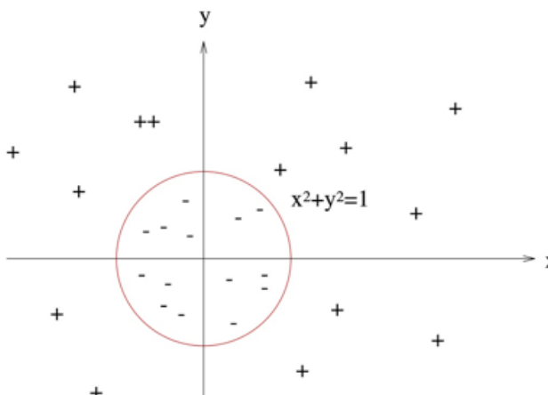
FIGURE 18: Exemple de transformation d'un cas non séparable (coordonnées cartésiennes) en cas séparable (coordonnées polaires). C'est un exemple trivial où les deux espaces ont la même dimension.
