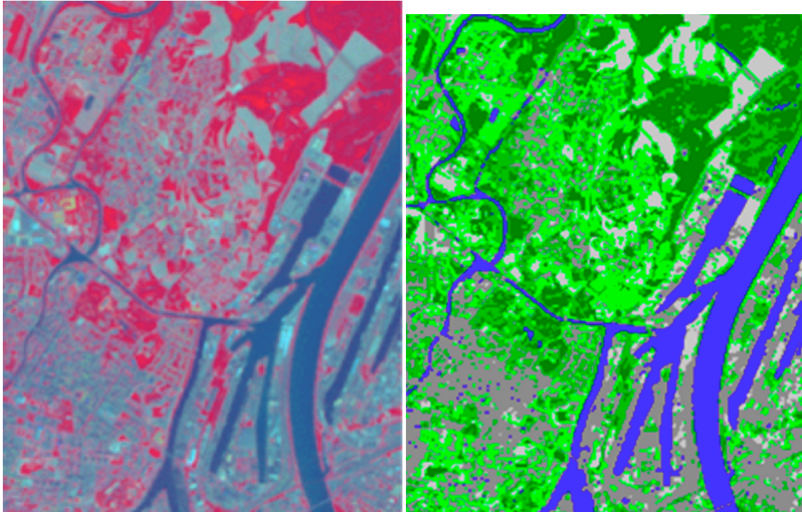
FIGURE 10: Exemple d'application du Kmeans sur une image SPOT. Gauche/A Image spot. Droite/B La même image avec 5 clusters colorés et identifiés par la méthode Kmeans.
