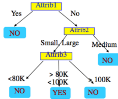
FIGURE 7: Arbre de décisions. Les nœuds (attributs) sont en jaune, les feuilles (classes) en bleu.
