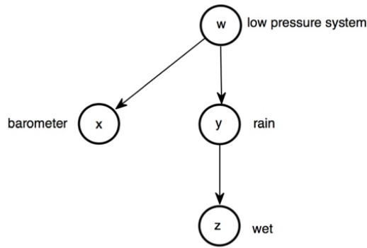
FIGURE 3: Graphe orienté du système x,y,z,w utilisé en exemple. Un arc allant d'un sommet A vers un sommet B signifie une forte probabilité que B soit la cause de A.
