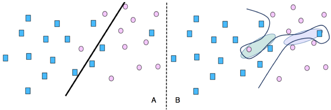
FIGURE 9: Illustration du cas de deux classes dont la séparation est non-linéaire. A/ Le plan (droite noire linéaire) est trop simple pour bien séparer les classes bleue et rose. C'est un cas de sous-ajustement aux données. B/ Le plan (courbe noire non linéaire) est très complexe. Même s'il sépare parfaitement les deux classes, il sera incapable de bien classer une nouvelle donnée apparaissant dans les régions verte ou bleue. C'est un cas de sur-ajustement aux données.
