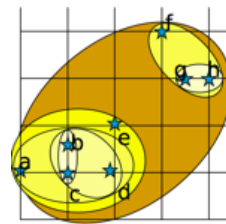
FIGURE 12: La CAH est achevée. La représentation hiérarchique permet a posteriori de choisir un nombre de clusters pertinents pour séparer les données. Ici, k=2 paraît intéressant. Le 1er cluster a les données f, g et h ; le 2nd les données e, a, d, b et c.
