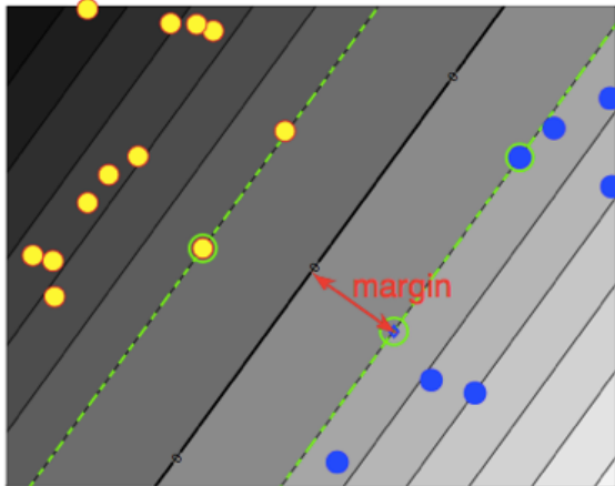
FIGURE 16: La marge. Illustration pour le cas séparable où toutes les données des deux classes peuvent être séparées par une droite (linéairement séparable).
