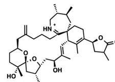
spirolide I
