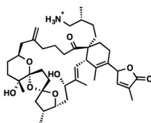
spirolide E
