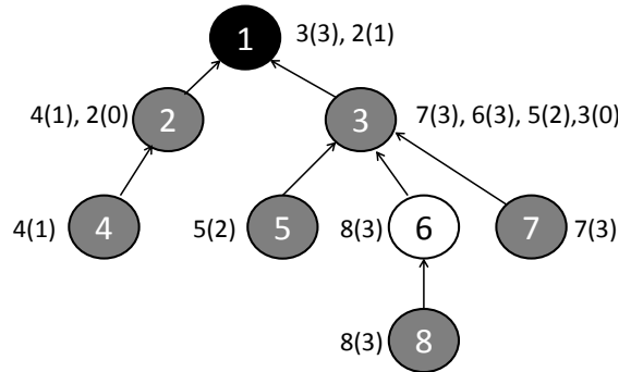
(d) End state with "Level-Distance" heuristic
