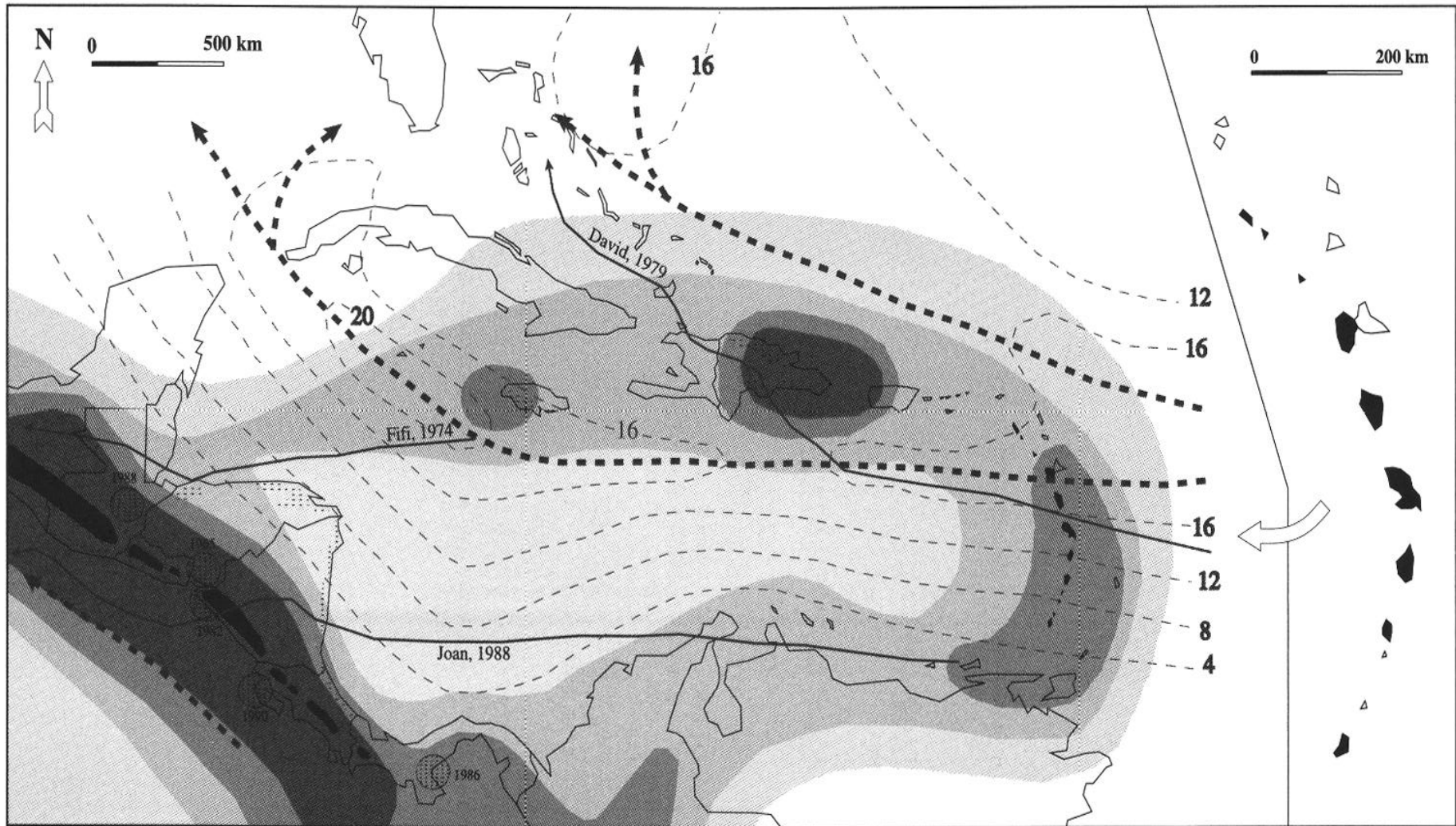
Fig. 1 Carte des aléas (Amérique Centrale et Caraïbe). Hazards map (Central America and the Caribbean).
