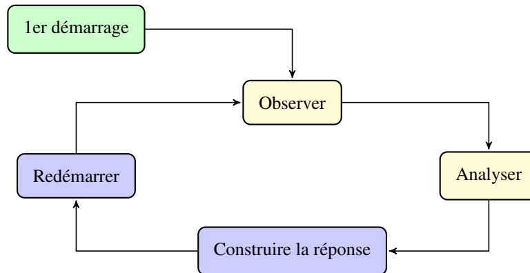
Figure 6. Méthode itérative
