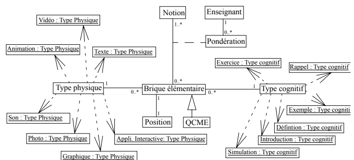
FIG. 5 - Représentation des briques élémentaires
