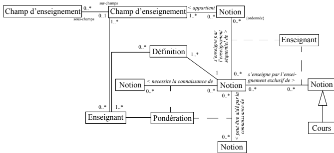
FIG. 2 - Primitives de construction du modèle du domaine
