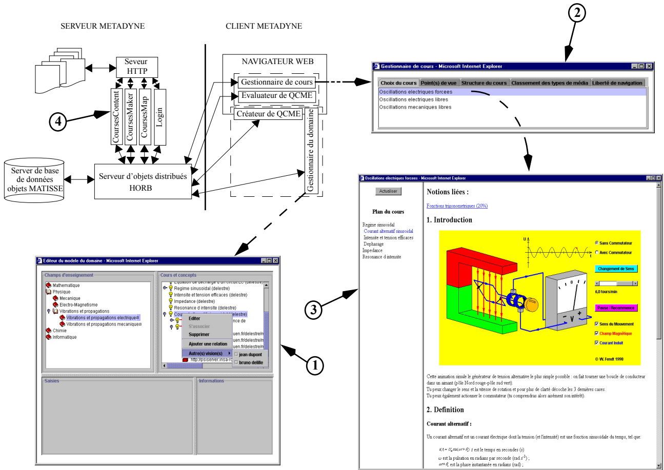
FIG. 8 - Architecture logicielle du prototype METADYNE
