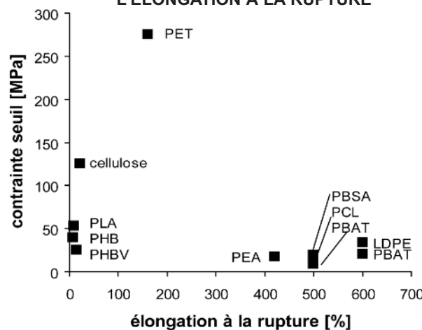
Figure 4 PROPRIÉTÉS MÉCANIQUES DES POLYMÈRES BIODÉGRADABLES EN COMPARAISON AVEC CELLES DES LDPE ET PET, CAS DE LA CONTRAINTE AU SEUIL ET DE L'ÉLONGATION À LA RUPTURE
