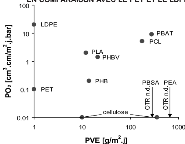
Figure 5. PROPRIÉTÉS BARRIÈRES À L'OXYGÈNE (TRANSMISSION OXYGÈNE, PO 2 ) ET À LA VAPEUR D'EAU (PERMÉABILITÉ À LA VAPEUR D'EAU, PVE) DE DIFFÉRENTS POLYMÈRES BIODÉGRADABLES EN COMPARAISON AVEC LE PET ET LE LDPE
