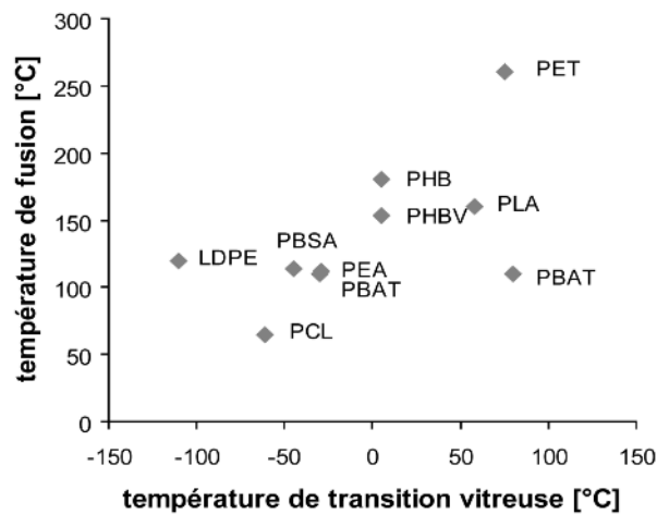
Figure 3 PROPRIÉTÉS THERMIQUES DE DIFFÉRENTES MATRICES POLYMÈRES MESURÉES À L'AIDE DE L'ANALYSE ENTHALPIQUE DIFFÉRENTIELLE
