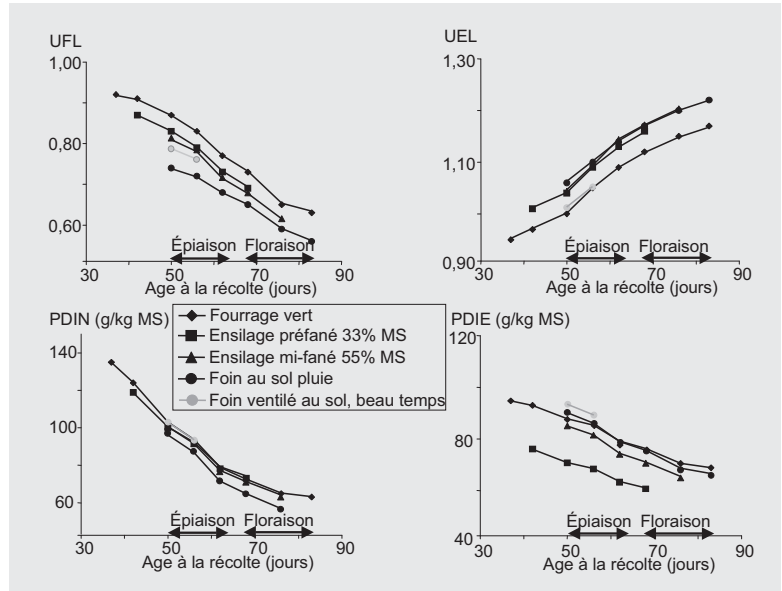
FIGURE 3 : Evolution de la valeur alimentaire du dactyle au premier cycle de végétation avec l'âge du fourrage à la récolte et le mode de conservation (données des Tables INRA, BAUMONT et al. , 2007b).
