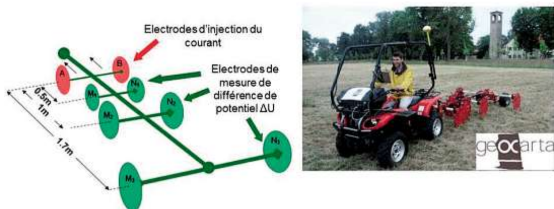
Figure 1 . Schéma et photographie du dispositif tracté ARP, déployé par la société GEOCARTA ( www.geocarta.net ). Photo : Geocarta.
