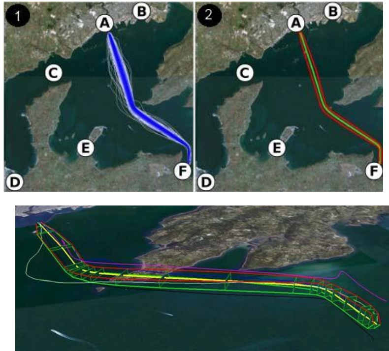
Figure 8. Agrégats de trajectoires de navires dans la rade de Brest en fonction des types de navires et de l'itinéraire (haut). Motif spatiotemporel représenté en 3D du cluster de trajectoires (bas). A B C D E et F sont des points de repère de l'espace support
