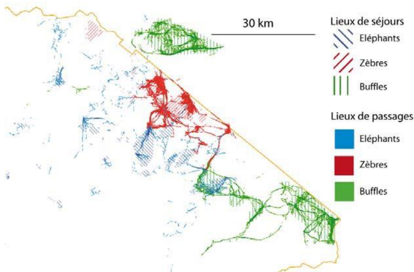
Figure 7. Lieux de fréquentation d'animaux par espèce
