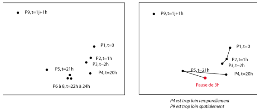
Figure 4. Exemple de filtrages physiques des positions numérotées de P1 à P9 : P4 et P9 ont été filtrés à cause de leur trop grande distance temporelle et spatiale des autres positions ; ils ne peuvent pas être atteints par l'objet mobile. Ils constituent deux trajectoires
