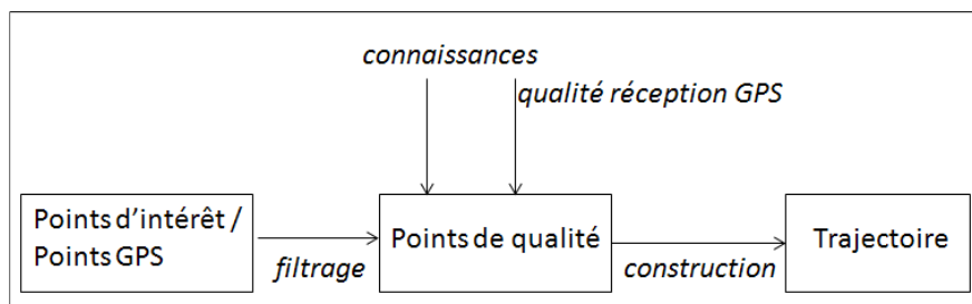
Figure 3. Étapes de filtres des positions puis de construction de trajectoire
