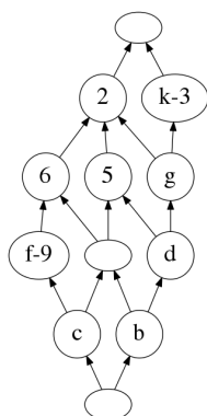
Figure 1: Un treillis avec ses noeuds irréductibles.
