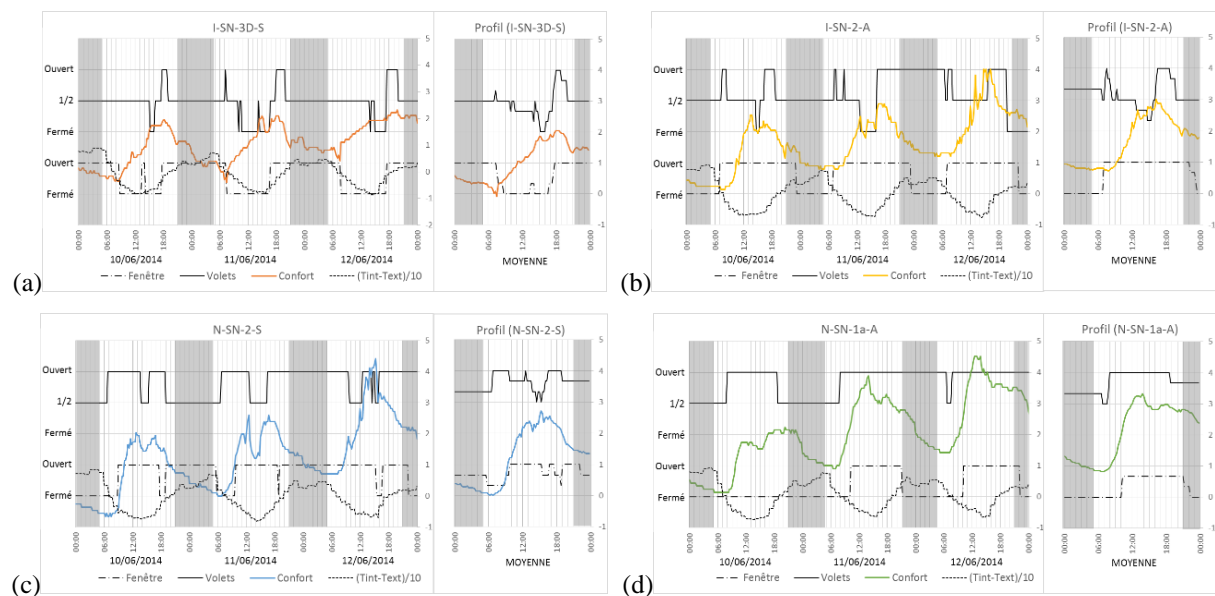
Figure 6. Écarts à la température de confort et position des fenêtres et des volets de quatre appartements sur trois jours du 10 au 12 juin 2014 et profils du comportement moyen de l’occupant sur les trois jours étudiés.
