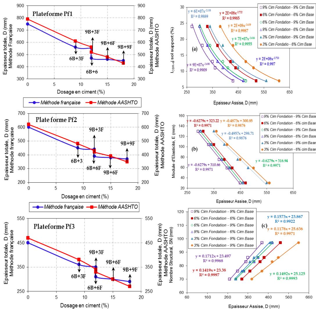
Figure 7. Evolution des épaisseurs en fonction de : (a, b et c) dosage dans les différentes couches, (d) I_{\text{CBR-4j}} , (e) E et (f) SN
