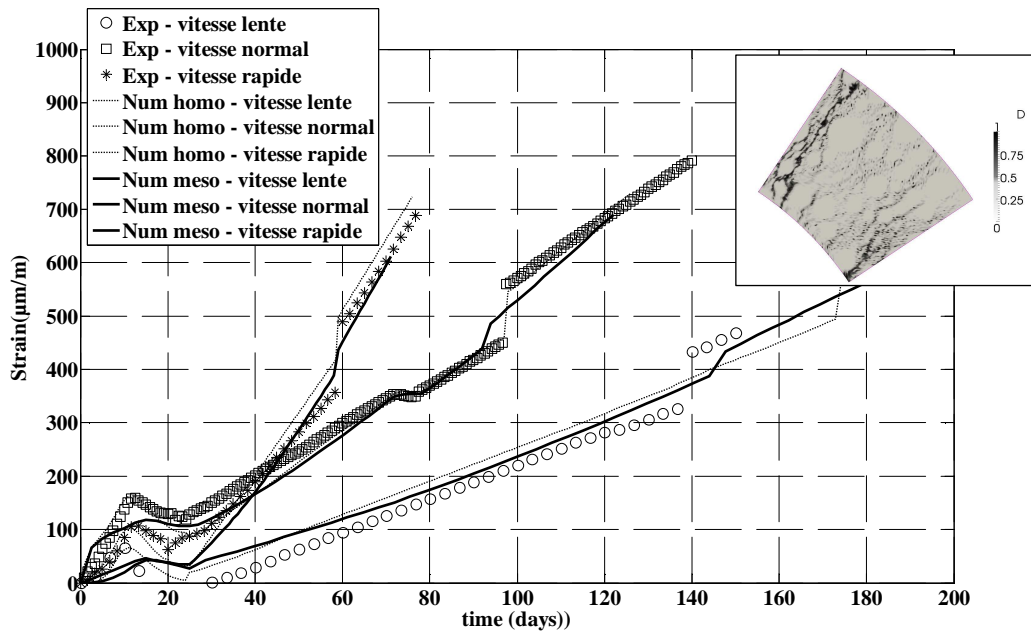
Figure 4 : Evolution des déformations des essais à l'anneau thermique actif : comparaison entre les mesures expérimentales, les prévisions d'un modèle macroscopique (homogène) et mésoscopique.
