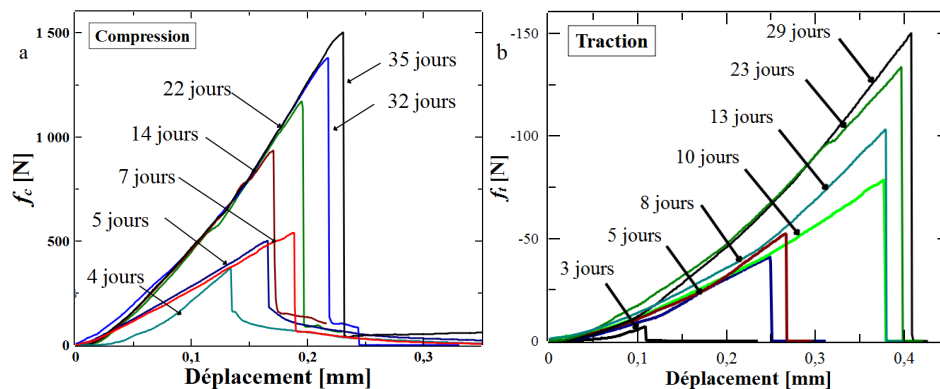
Figure 4. Courbes force - déplacement lors des essais de compression (a) et de traction (b).
