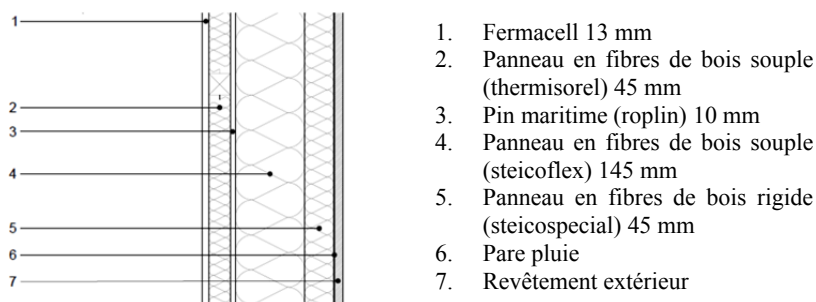
Figure 4. Composition de la paroi
