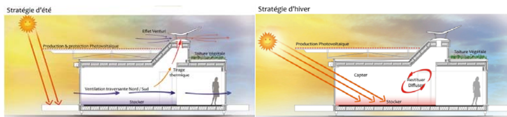
Figure 2. Stratégies de ventilation et de chauffage pendant la journée en été (en haut) et en hiver (en bas)
