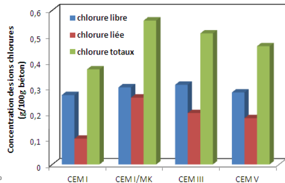
Figure 10. Teneur en chlorures liés, libres et totaux des BAP
