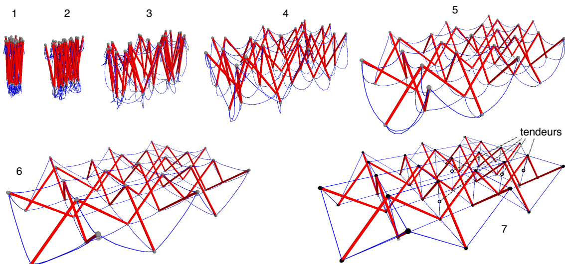
Figure 5. Étapes du déploiement (1 à 6) et état géométrique final atteint par ajout de tendeurs verticaux (7).
