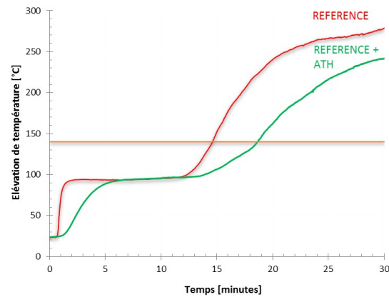
Figure 8. Influence de l'ajout d'ATH sur l'isolation au feu des sandwiches
