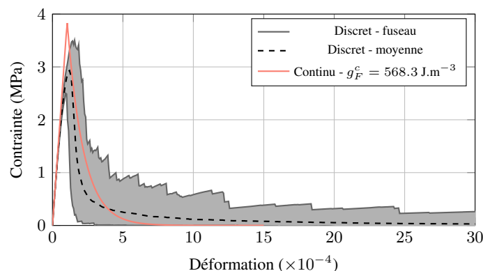
Figure 2 – Réponses en traction des modèles continus et discret.
