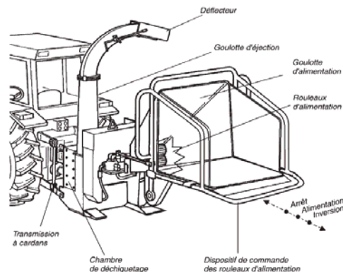
Figure 3: Principaux composants de la déchiqueteuse forestière [source: fiche sécurité machines agricoles et forestières -Irstea]
