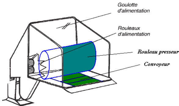
Figure 5: Solution de conception d'une déchiqueteuse à convoyeur et rouleau presseur
