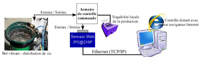
Figure 3. Traçabilité d'un sous ensemble sur une ligne de production via une solution Internet
