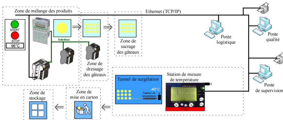
Figure 4. Installation sur une ligne de produits
