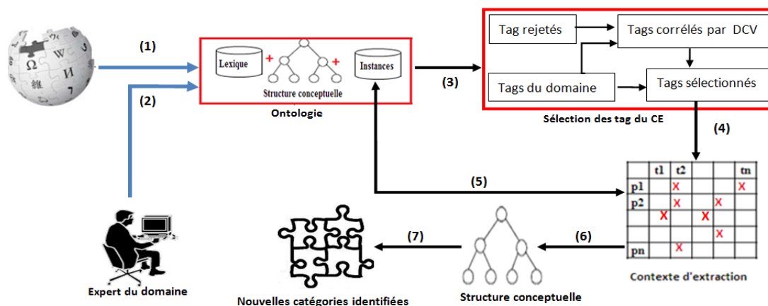
FIGURE 3 – Approche de découverte de nouvelles catégories dans un wiki sémantique.
