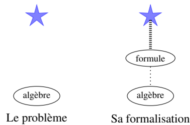
FIGURE 9. Un enchaînement pour représenter une approche algébrique
