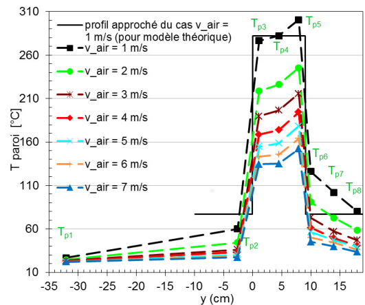
Figure 3 : Profils de température le long de la paroi de la conduite mesurés par les thermocouples T_{pi} ( i=1 à 8) (cf. Fig. 2), dans le cas de la tension de chauffage U_{max} = 24 V, pour différentes vitesses de l'air, v_{air} , en présence du bouclier vertical. L'approximation du profil de température pariétal par un profil symétrique en créneau pour le modèle théorique est illustré dans le cas v_{air} = 1 m/s.
