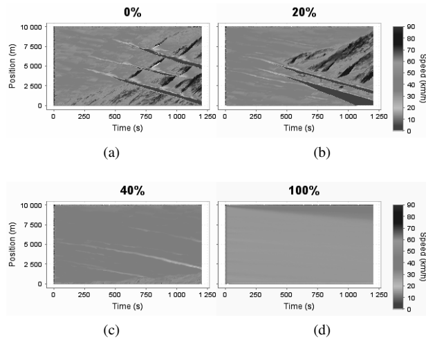
FIGURE 4 – Trajectoires et vitesses sur la voie de droite, pour plusieurs fractions de véhicules connectés parmi des véhicules non connectés (a : 0%, b : 20%, c : 40% et d : 100%).
