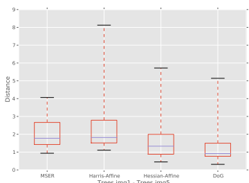
(d) Trees img1 - img5.
