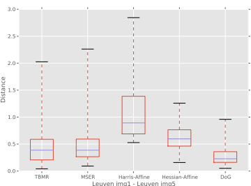
(d) Leuven img1 - img5.
