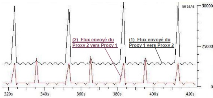
FIGURE 13: Courbes du trafic échangé entre les deux proxies DDS
