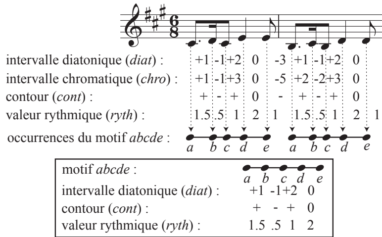
FIG. 1.2 – Description de la partition suivant différentes dimensions musicales. Les deux motifs encadrés sont deux occurrences d’un motif abcde de description diat = (+1, -1, +2, 0) , cont = (+, -, +, 0) et ryth = (1.5, 0.5, 1, 2) .
