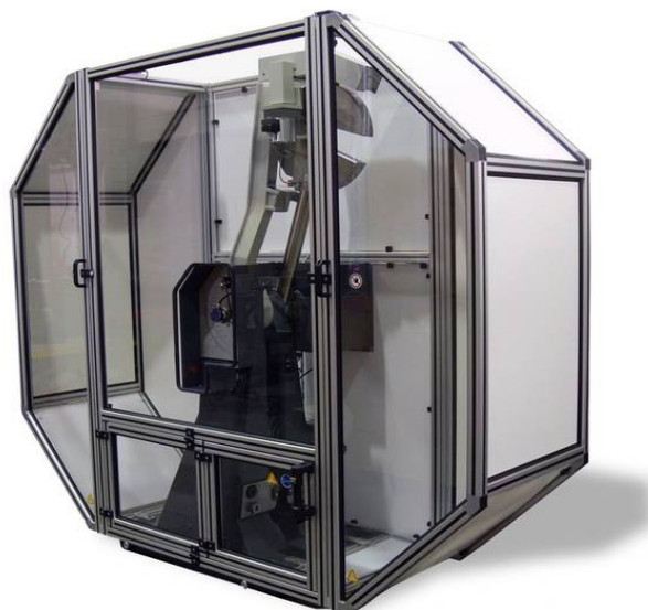
Mouton de Charpy 750 joules, dispositif utilisé pour la mesure de la résilience des aciers (tiré du cours Produits Procédés et Matériaux de X. Pessoles 2013)
