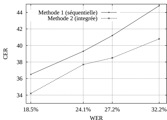
FIG. 2: Évolution du CER en fonction du WER
