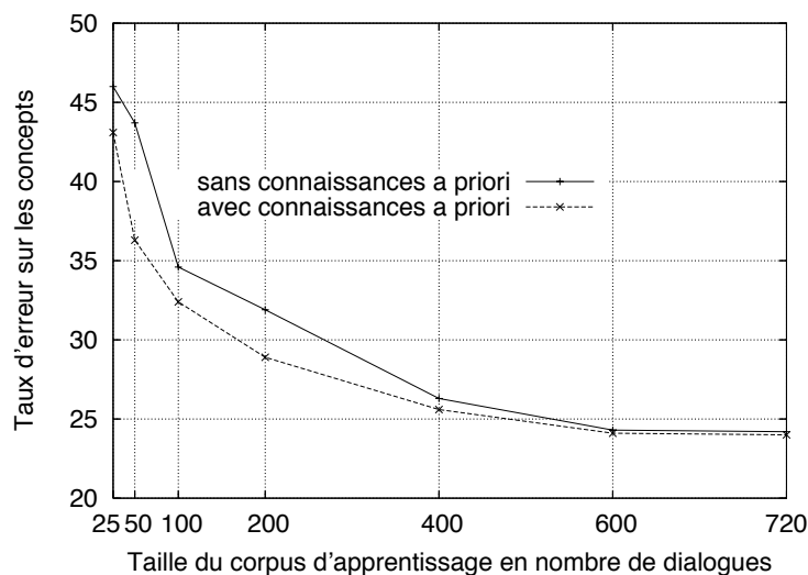
Figure 1. Taux d'erreur sur les concepts en fonction de la taille du corpus d'apprentissage, avec et sans connaissances a priori
