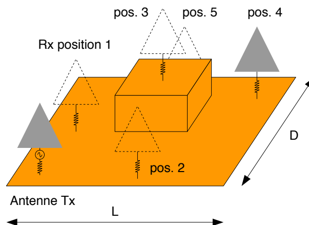
Figure 1. Transmission entre antennes ULB : la position de l'antenne de réception varie.
